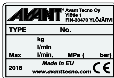
Redskapets identifikasjonsplate A442056 / A442032 / A440869
